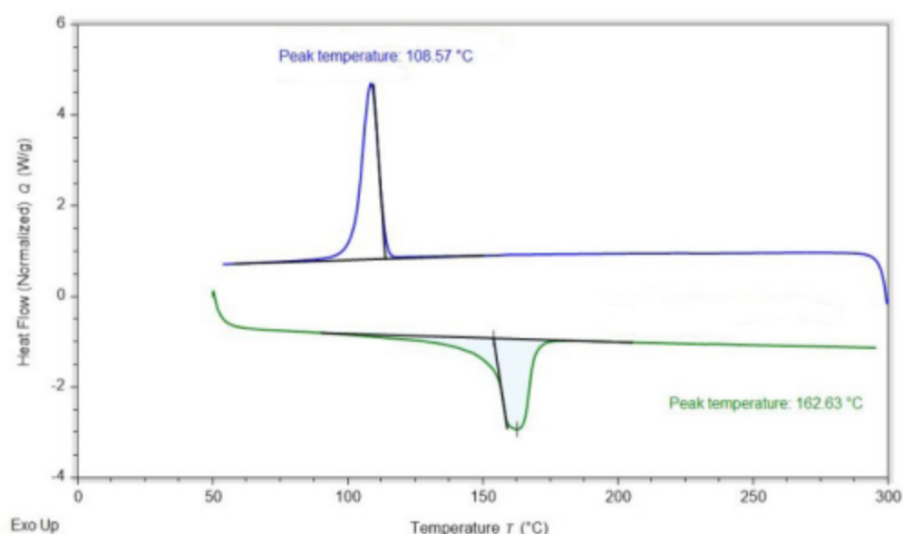
图 C.1 聚丙烯长丝纺粘非织造土工布熔点参考测试图谱
