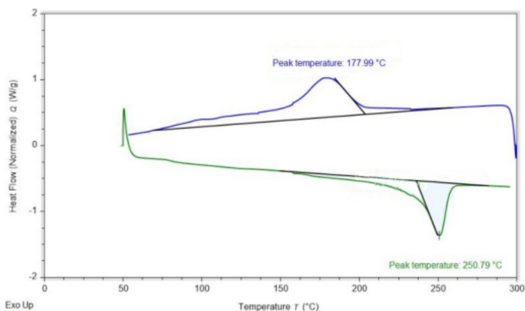
图 C.2 聚酯长丝纺粘非织造土工布熔点参考测试图谱
