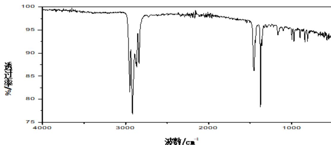
图 A.1 聚丙烯长丝纺粘非织造土工布红外光谱参考测试图谱
